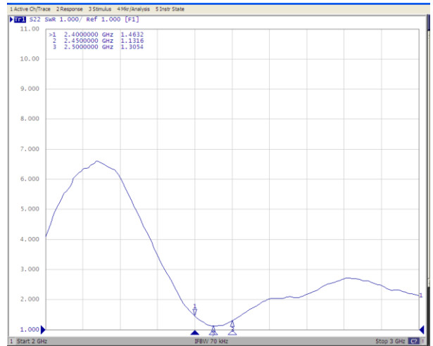
V.S.W.R
