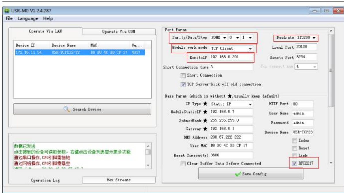
Diagram 5.1.1-4 Serial parameters
