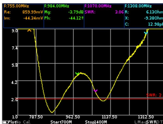
Рисунок 10.8 – График КСВН
