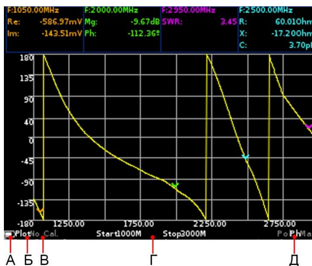
Рисунок 8.1 – Экран прибора
