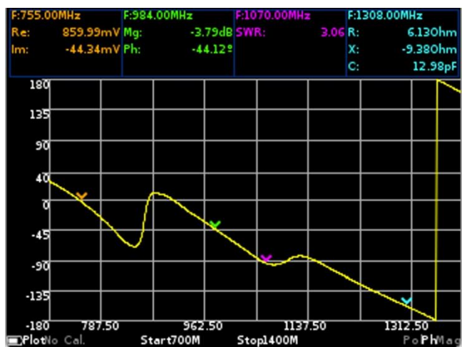
Рисунок 10.3 – График фазы
